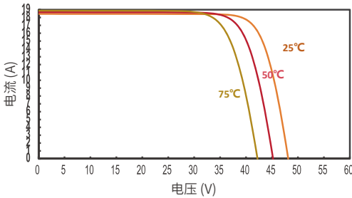
JT715SLk(B) 不同温度下的IV曲线
