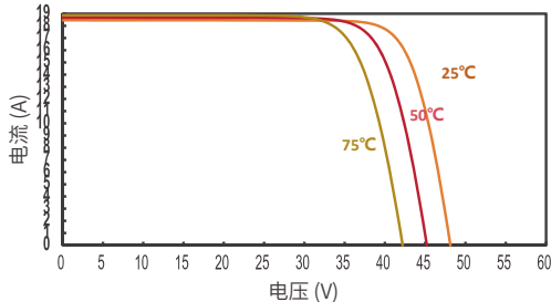
JT715SLk(B) 不同温度下的IV曲线
