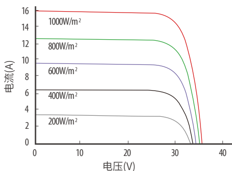
JT445Snt(B) 不同光强下的IV曲线 电池片温度 25°C
