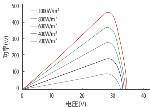
JT445Snt(B) 不同光强下的PV曲线
