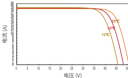
JT730SLk(B) 不同温度下的IV曲线
