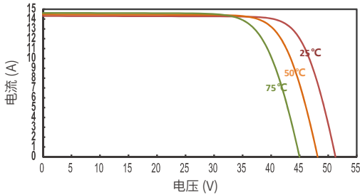
JT570SSt(B) 不同温度下的IV曲线
