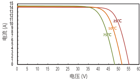
JT610SRt(B) 不同温度下的IV曲线
